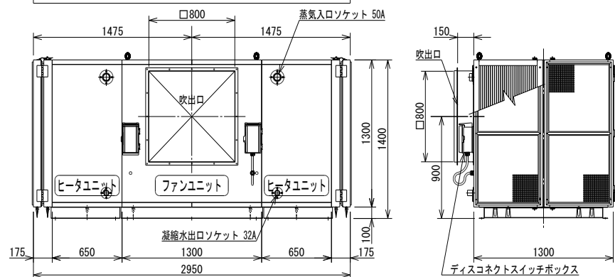
CSFH-7137S1-E3 / CSFH-7155S1-E3
