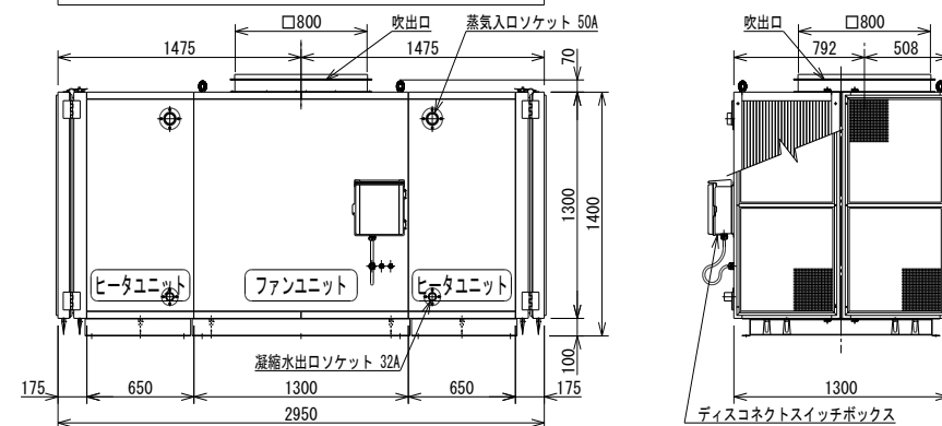
CSFH-7137U1-E3 / CSFH-7155U1-E3
