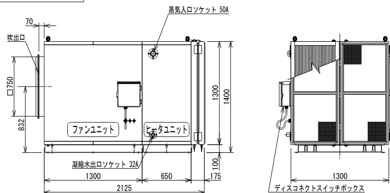
CSFH-6322S-E3
