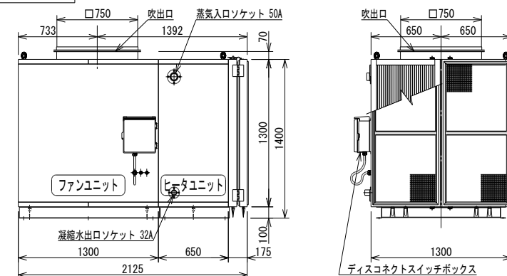
CSFH-6322U-E3
